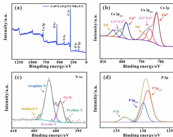
Fig. 3 (a) XPS spectrum, (b) Co 2p, (c) N 1s, and (d) P 2p of \text{CoP}/\text{CoN}@\text{NCNRs}/\text{CC} .
