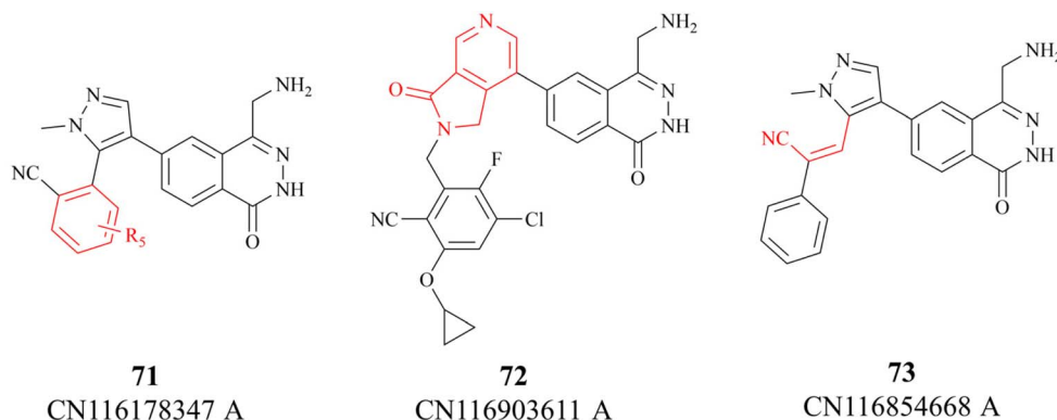
Fig. 8 27 (MRTX1719) analogues.
