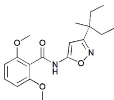
Isoxaben
