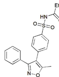
Parecoxib
