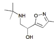
Broxaterol
