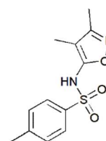
Sulfisoxazole
