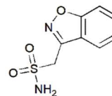
Zonisamide
