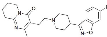
Risperidone
