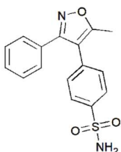
Valdecoxib
