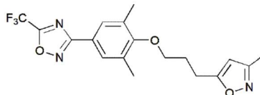
Pleconaril
