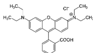
Rhodamine 6G
