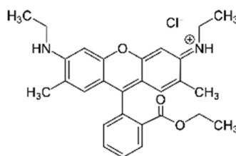
Rhodamine 6G
