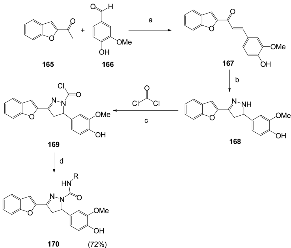
a: ZrCl 4 , DCM, RT, 1 h. b: NH 2 NH 2 ·H 2 O, ETOH/reflux. 3. h c: TEA, dry THF, RT, 4 h. d: K 2 CO 3 , DCM, N 2 atm, 3-5 h. R-NH 2 .
