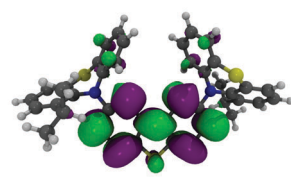
LUMO
