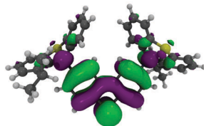
HOMO
