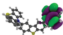
HOMO
