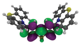
LUMO
