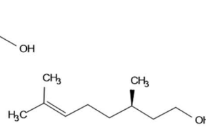
Geraniol
