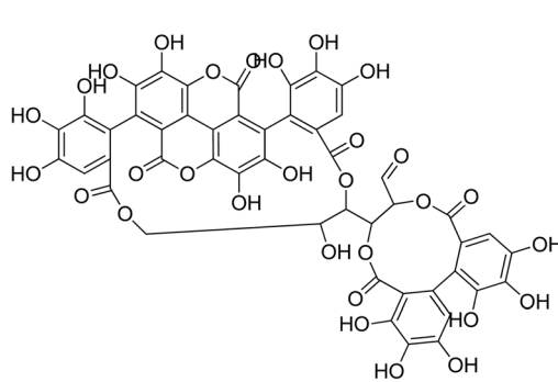
Punicalagin
