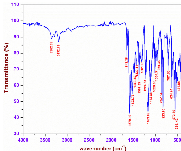
Fig. 3 FTIR spectrum of DMMA.
