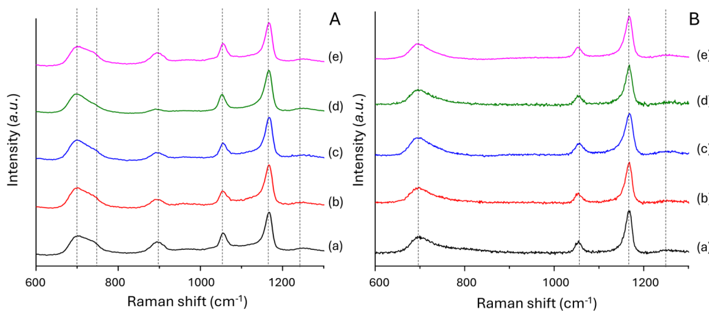
Fig. 6 Raman spectra of (A): (a) PGP-Mn0; (b) PGP-Mn1; (c) PGP-Mn3; (d) PGP-Mn5; (e) PGP-Mn10 and (B): (a) PGF-Mn0; (b) PGF-Mn1; (c) PGF-Mn3; (d) PGF-Mn5; (e) PGF-Mn10.
