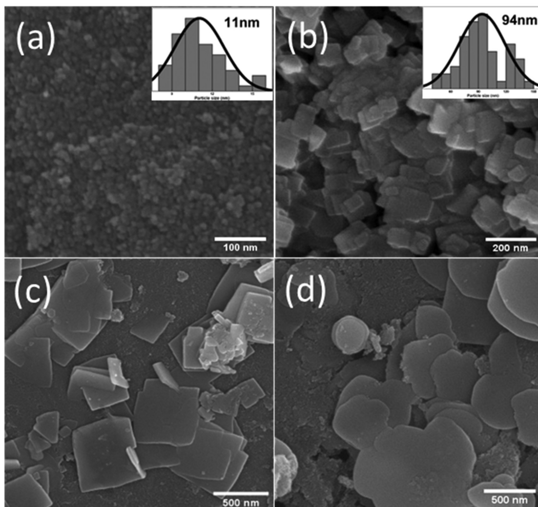
Fig. 3 FESEM images of (a) \text{SnO}_2 , (b) \text{BiOBr} (c) \text{SnO}_2\text{-BiOBr} , (d) \text{SnO}_2\text{-BiOBr-rGO} .
