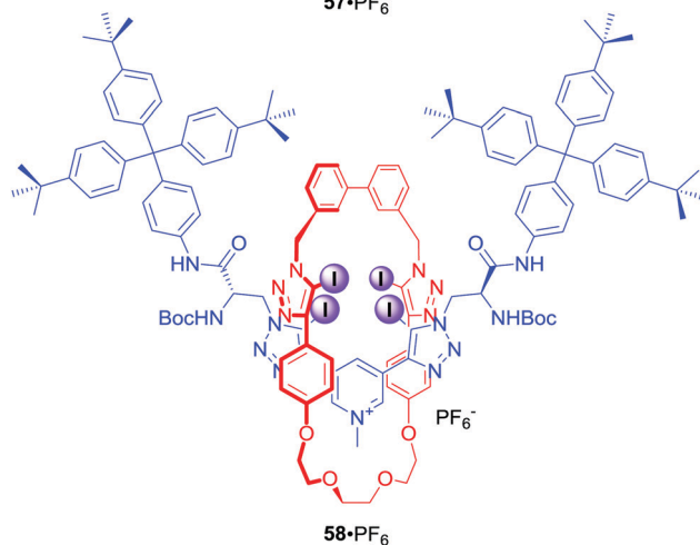
Fig. 26 Chiral XB [2]rotaxanes.
