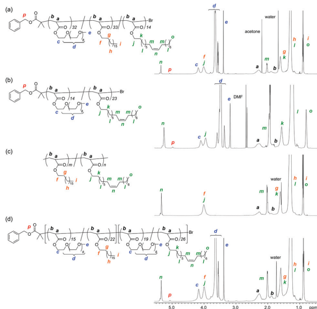
Fig. 3 ^1\text{H} NMR spectra of (a) P4 , (b) P7 , (c) P8 , and (d) P9 in \text{CDCl}_3 at 25\text{ }^\circ\text{C} .
