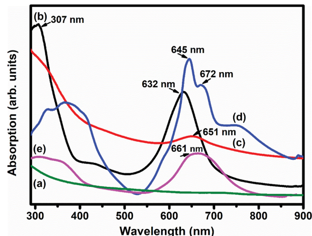
Fig. 5 UV-vis absorption spectra of (a) SWCNTs-COOH; (b) F_{16}CoPc ; (c) S_1 ; (d) F_{16}ZnPc and (e) the S_2 hybrid.
