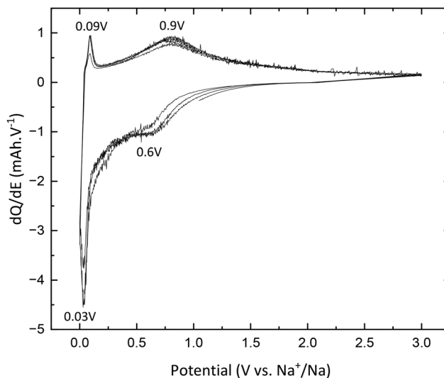
Fig. 12 dQ/dE curves of \text{TiO}_2 @C.
