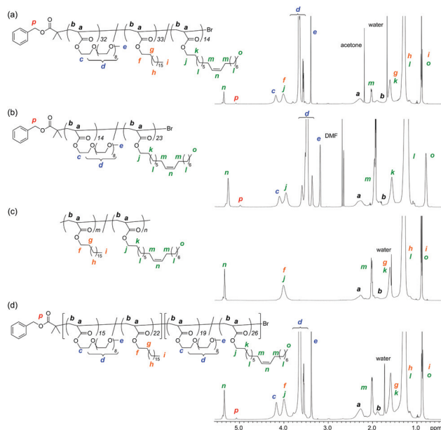
Fig. 3 ^1\text{H} NMR spectra of (a) P4 , (b) P7 , (c) P8 , and (d) P9 in \text{CDCl}_3 at 25\text{ }^\circ\text{C} .
