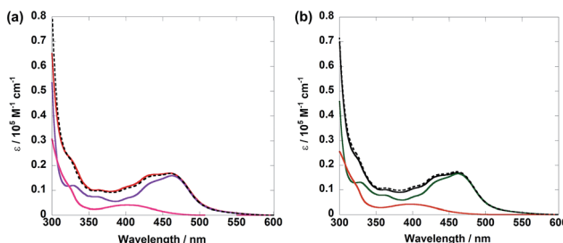
Fig. 1 UV-vis absorption spectra of (a) Ru(CH 2 OCH 2 )Re (red), Ru(CH 2 OCH 2 ) (purple), and Re(CH 2 OCH 2 ) (pink), and Ru(CH 2 OCH 2 ) (black), Ru (green), and Re (red). The dotted lines show the 1:1 summation spectrum of (a) Ru(CH 2 OCH 2 ) and Re(CH 2 OCH 2 ) and (b) Ru and Re . Dimethylformamide (DMF) was used as the solvent.
