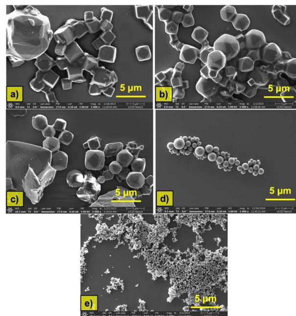
Fig. 4 SEM Images of: (a) Zn-poly(OCTbdc-5a) 35 , (b) Zn-tBu-poly(OCTbdc-5a) 29 , (c) Zn-Py-poly(OCTbdc-5a) 29 , (d) Zn-PS 12 - block -poly(OCTbdc-5a) 23 - block -PS 12 , and (e) Zn-PS 30 - block -poly(OCTbdc-5a) 23 - block -PS 30 .
