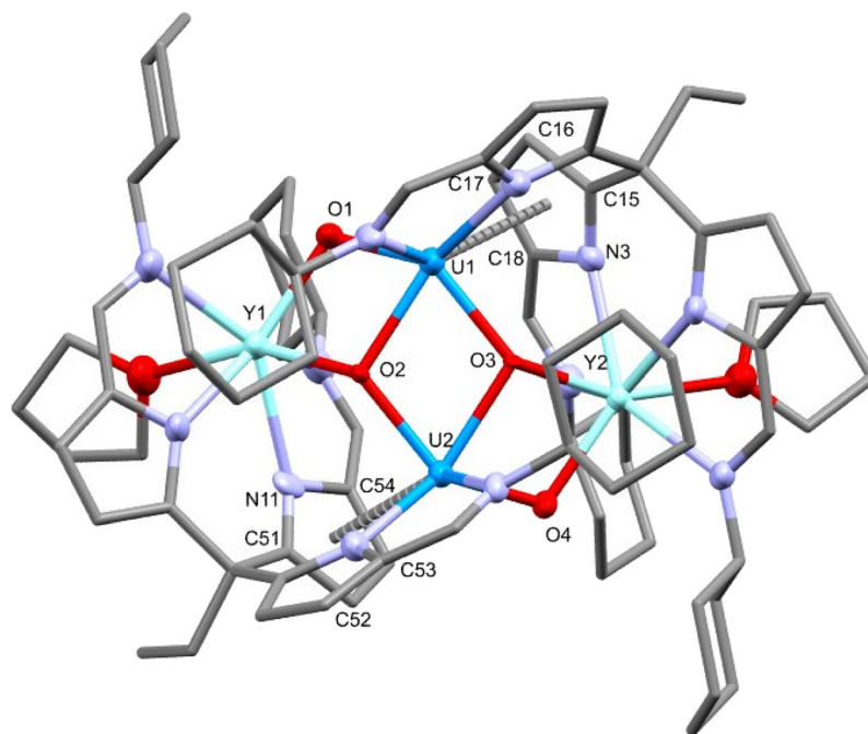
Complex U1-O1 U1-O2 RE1-O1 U1-RE1 O1-U1-O2 U1-O1-RE1 6-Y' 1.951(2) 1.852(2) 2.242(2) 3.7979(6) 179.2(1) 129.8(1) 6-Dy' 1.939(2) 1.849(3) 2.268(3) 3.7876(6) 179.2(1) 128.2(2)
