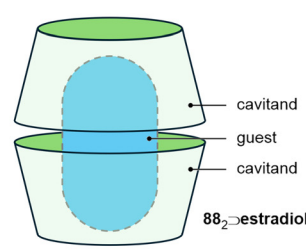
Estradiol
