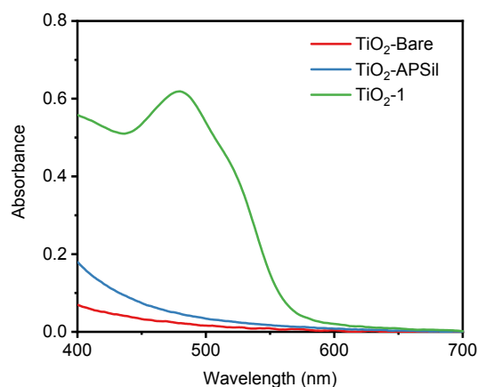
Fig. 1. UV-Vis spectra comparing the solid-state absorption spectra of TiO 2 -Bare, TiO 2 -APSil and TiO 2 -1.
