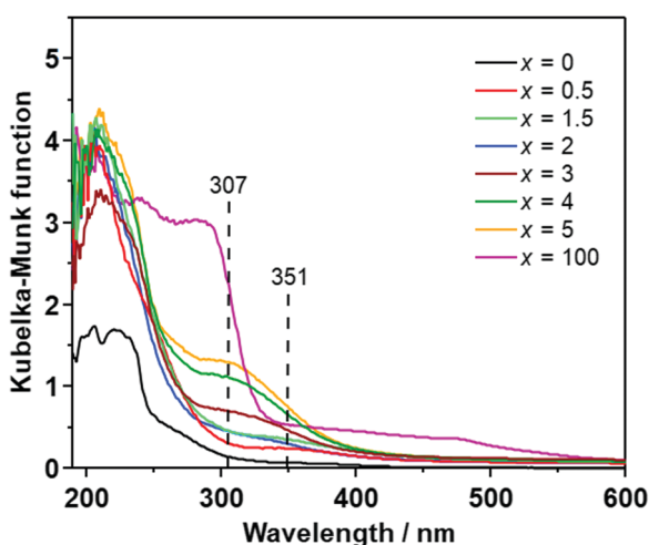
Fig. 2 UV-Vis spectra of \text{Li}_2\text{S} ( x = 0 ), \text{AlI}_3 ( x = 100 ), and (100 - x)\text{Li}_2\text{S}\cdot x\text{AlI}_3 .
