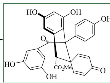
(-)-245: Hopeanol
