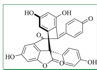
(-)-244: Hopeahainol A
