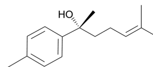
Fig. 12 (+)-(R)-Gossonorol.
