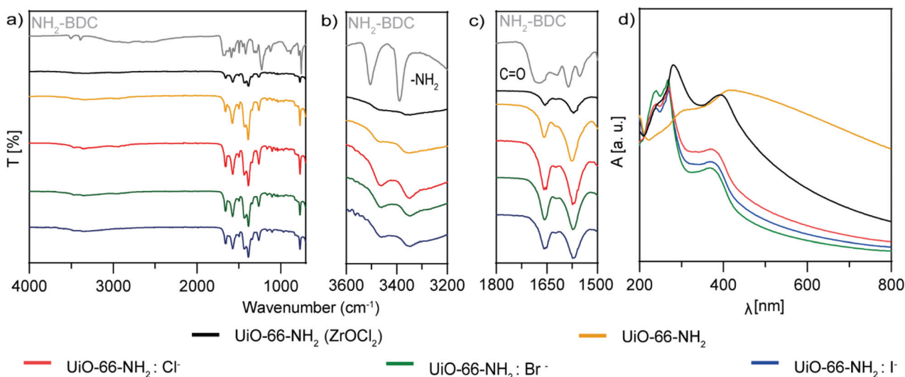
Fig. 4 (a–c) FTIR analysis and (d) UV-vis spectroscopy of UiO-66-NH 2 NMOFs: UiO-66-NH 2 (ZrOCl 2 ) (black), UiO-66-NH 2 (orange), UiO-66-NH 2 : Cl - (red), UiO-66-NH 2 : Br - (green) and UiO-66-NH 2 : I - (blue).
