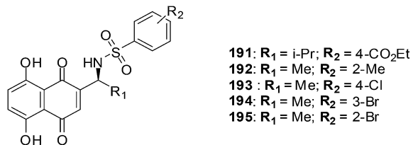
Fig. 39 Shikonin analogues.
