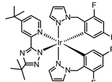
Ir(dfb-pz) 2 (bbptz) 53
