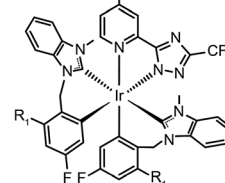
55: R 1 = H, R 2 = t Bu (fbmb) 2 Ir(bptz)
