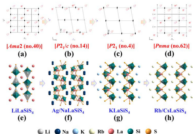
Fig. 3 Structural fluctuations in A^I\text{LaSiS}_4 ( A^I = \text{Li, Ag, Na, K, Rb, Cs} ): (a–d) symmetry changes from Ama2 ( \text{LiLaSiS}_4 ), P2_1/c ( \text{AgLaSiS}_4/\text{NaLaSiS}_4 ), and P2_1 ( \text{KLaSiS}_4 ) to Pnma ( \text{RbLaSiS}_4 and \text{CsLaSiS}_4 ); (e–h) the crystal structures of \text{LiLaSiS}_4 (e), \text{Ag/NaLaSiS}_4 (f), \text{KLaSiS}_4 (g), and \text{Rb/CsLaSiS}_4 (h).
