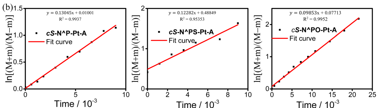
Fig. 8 (a) X-ray single-crystal structures, dihedral angles, and experimental interconversion energy barriers of cS-N1 O -Pt-A, cS-N2 O -Pt-B, cS-N P -Pt-A, cS-N PO -Pt-A, and cS-N PS -Pt-A; (b) investigation of rotation barriers of cS-N P -Pt-A, cS-N PO -Pt-A, and cS-N PS -Pt-A.
