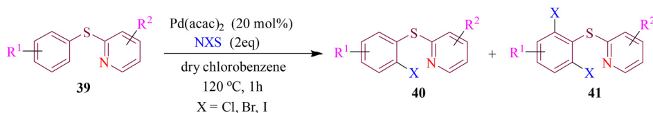
ortho -halogenation
