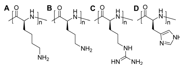
Fig. 3 Chemical structures (A) poly(L-lysine), (B) poly(L-ornithine), (C) poly(L-arginine), (D) poly(L-histidine).
