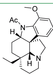
134 : (-)-Aspidospermine
