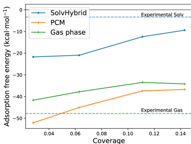
(a) Benzene
