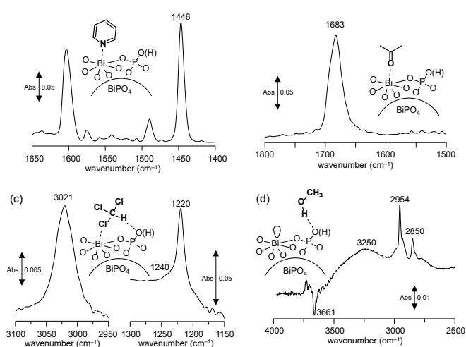
Fig. 8 Difference IR spectra for (a) pyridine-, (b) acetone-, (c) chloroform-, and (d) \text{CH}_3\text{OH} -adsorbed \text{BiPO}_4 -DEG at 25^\circ\text{C} .
