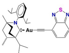
Au2 , quadrupolar A-Au-D-Au-A 2PA chromophore
