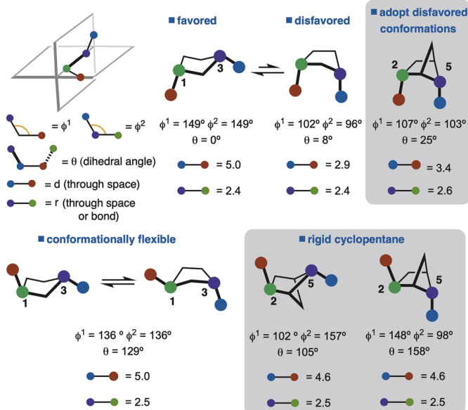
Fig. 1 Bicyclo[2.1.1]hexanes.
