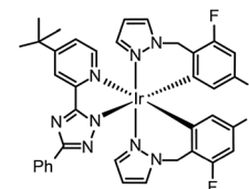
Ir(dfb-pz) 2 (bbptz) 52
