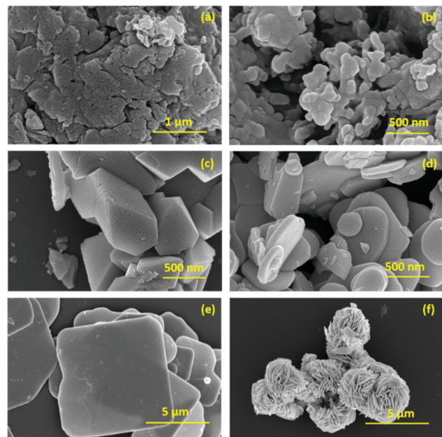
Fig. 3 FESEM images of (a and b) g-C 3 N 4 , (c) BiOF, (d) BiOCl, (e) BiOBr and (f) BiOI.
