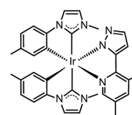
(mpmi) 2 Ir(dmpypz)
