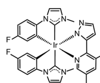
(fpmi) 2 Ir(dmpypz)
