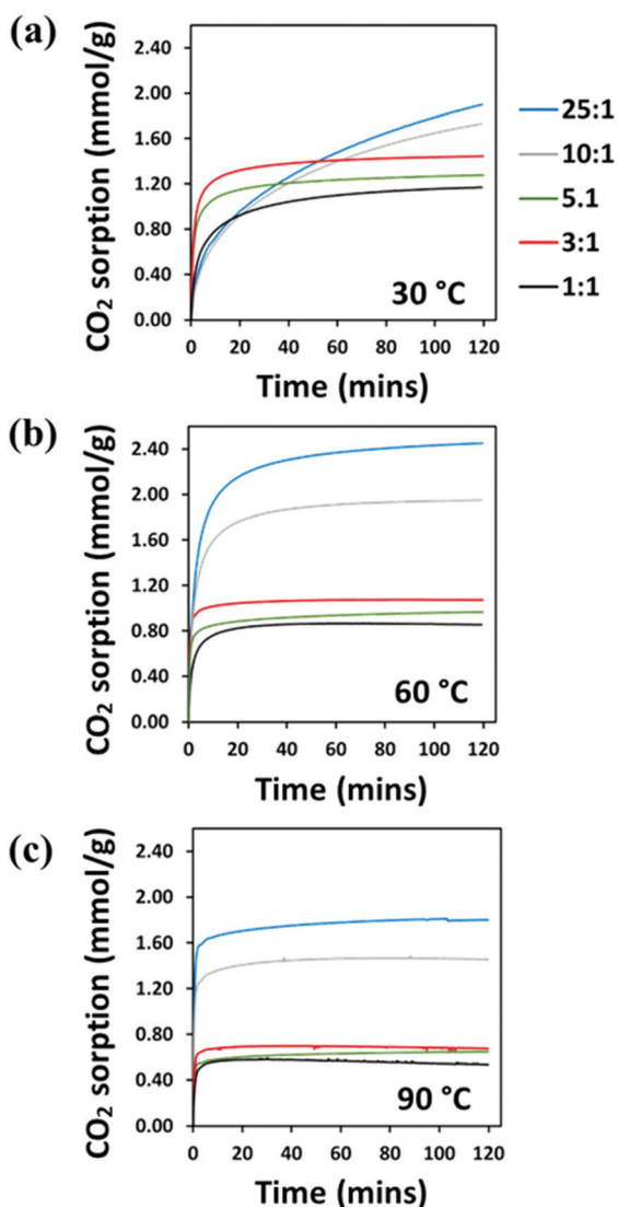
Fig. 7 TGA- \text{CO}_2 sorption ( \text{mmol g}^{-1} ) of PEI-4BMFPT 1 : 1 (V), 3 : 1 (V), 5 : 1 (V), 10 : 1 (V), 25 : 1 (V) at (a) 30 °C; (b) 60 °C; (c) 90 °C, under 90% \text{CO}_2 .
