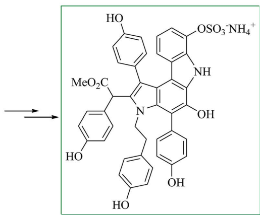
275: Dictyodendrin
