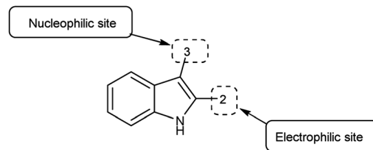
Fig. 21 Indole.
