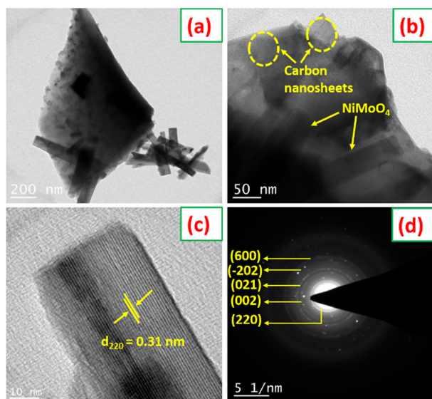
Fig. 6 (a)–(d) HRTEM images of \text{NiMoO}_4/\text{C} (D50) with the SAED pattern.
