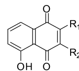
Juglone: R_1 = R_2 = H
