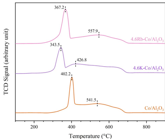
Fig. 9 H_2 -TPR profiles of Co/Al_2O_3 , 4.6K- Co/Al_2O_3 , and 4.6Rb- Co/Al_2O_3 catalysts.
