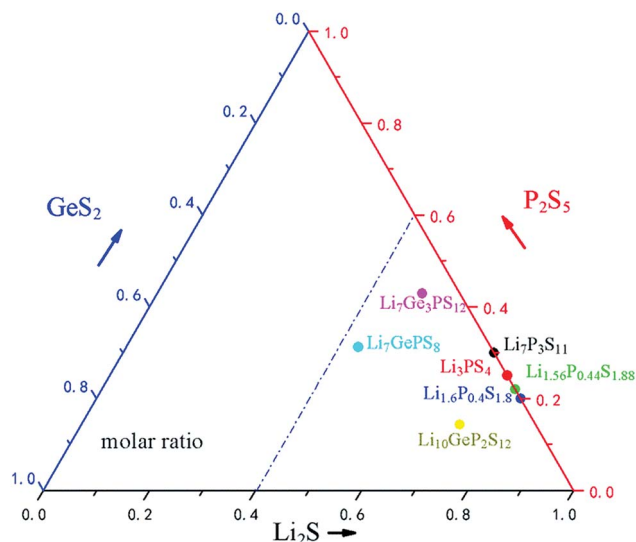
Fig. 5 \text{Li}_2\text{S} - \text{P}_2\text{S}_5 - \text{GeS}_2 ternary phase diagrams.
