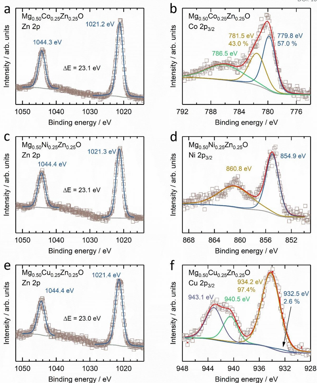
Fig. 3. XPS results of (a, c, e) Zn 2p and (b) Co 2p 3/2 , (d) Ni 2p 3/2 and (f) Cu 2p 3/2 of (a, b) Mg 0.50 Co 0.25 Zn 0.25 O, (c, d) Mg 0.50 Ni 0.25 Zn 0.25 O and (e, f) Mg 0.50 Cu 0.25 Zn 0.25 O.
