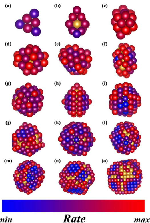
Fig. 6 Schematics of the reaction rate of CO oxidation on all surface sites of sub-nano-Au clusters, including (a) Au 6 , (b) Au 19 , (c) Au 25 , (d) Au 35 , (e) Au 53 , (f) Au 55 , (g) Au 73 , (h) Au 77 , (i) Au 112 , (j) Au 140 , (k) Au 159 , (l) Au 199 , (m) Au 234 , (n) Au 293 and (o) Au 300 .
