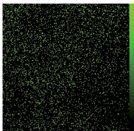
O Ka
