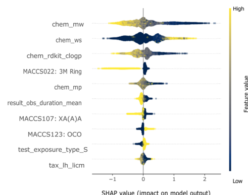
(d) Local SHAP values.
